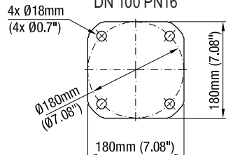
Размеры фланца устройства DN 100 PN16
