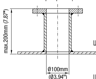
Размеры фланца емкости
